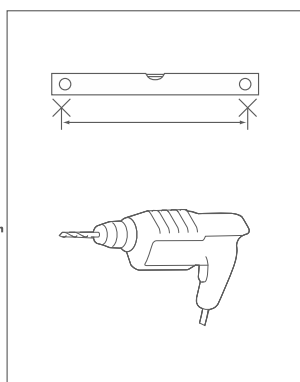
Rozstawy otworów dla poszczególnych grzejników
