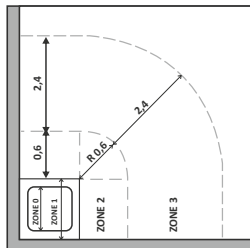
BEISPIEL FÜR DIE KLASSIFIZIERUNG VON BEREICHEN IN RÄUMEN MIT DUSCHEN
